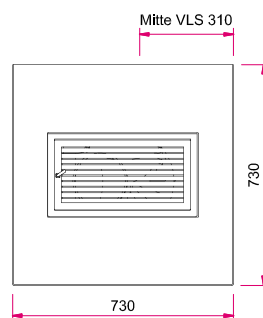
Draufsicht M 1:25
