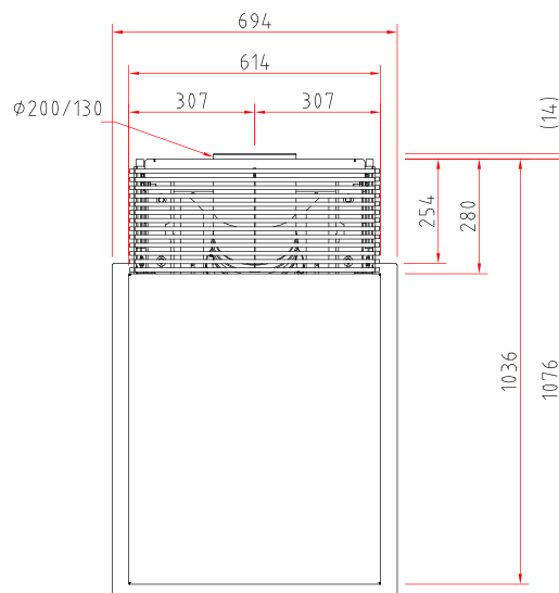
Draufsicht M 1:20
