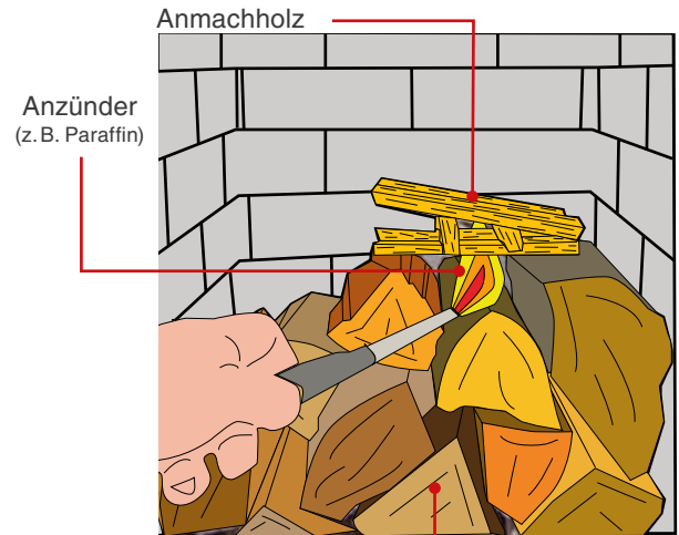
Abb. 6.1 Beispiel: Anzündvorgang
