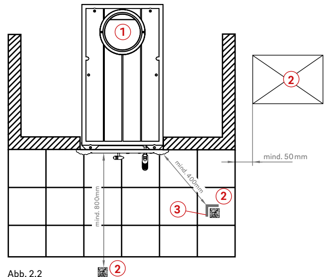
Abb. 2.2 Beispiel: Brennbarer Gegenstände und Strahlungsschutz
