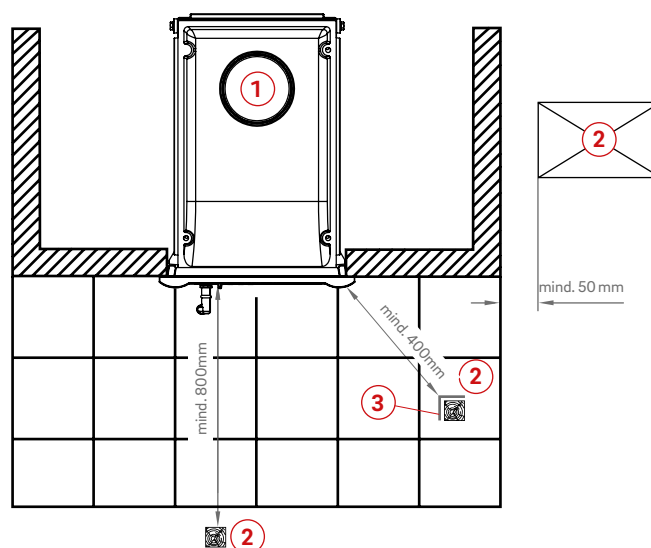
Abb. 2.2 Beispiel: Brennbare Gegenstände und Strahlungsschutz 1 = Heizeinsatz, 2 = z. B. Möbelstück, 3 = Strahlungsschutz
