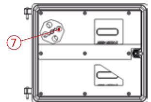
Innenansicht Aschetür
