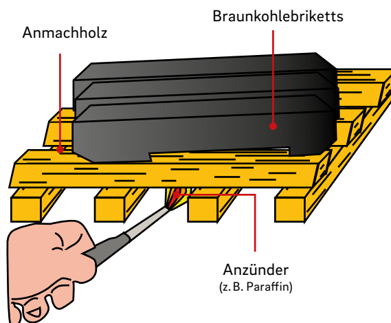
Abb. 8.1 Beispiel: Anzündvorgang
