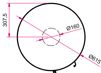
Draufsicht M 1:20
