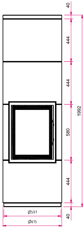
Frontansicht M 1:20
