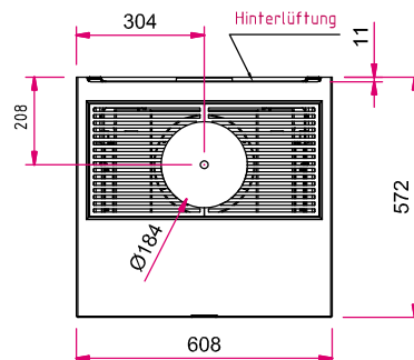
Draufsicht M 1:20
