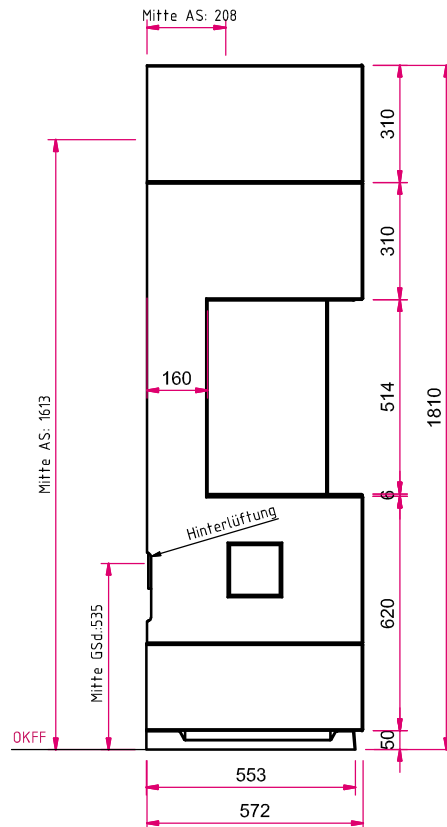
Seitenansicht links M 1:20
