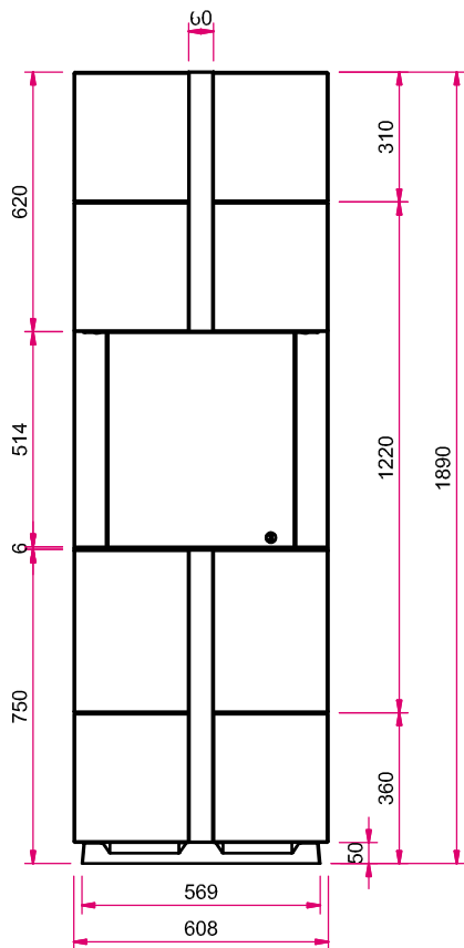
Frontansicht M 1:20
