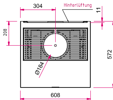
Draufsicht M 1:20
