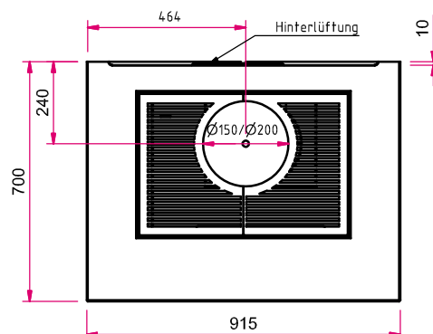
Draufsicht M 1:20
