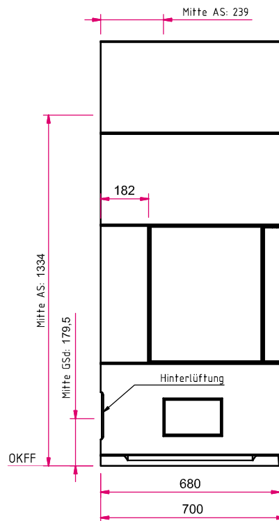
Seitenansicht links M 1:20
