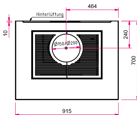
Draufsicht M 1:20
